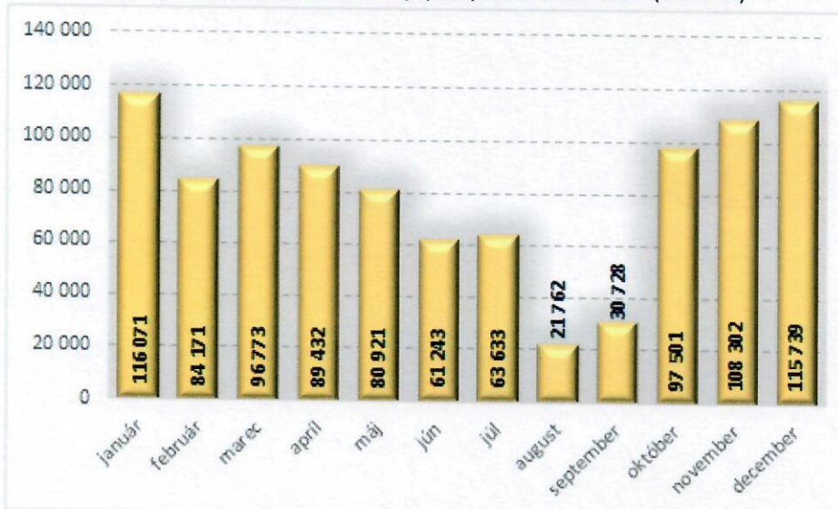
PPC Energy, a.s.: Spotreba zemného plynu počas roka 2017 (v MWh)
