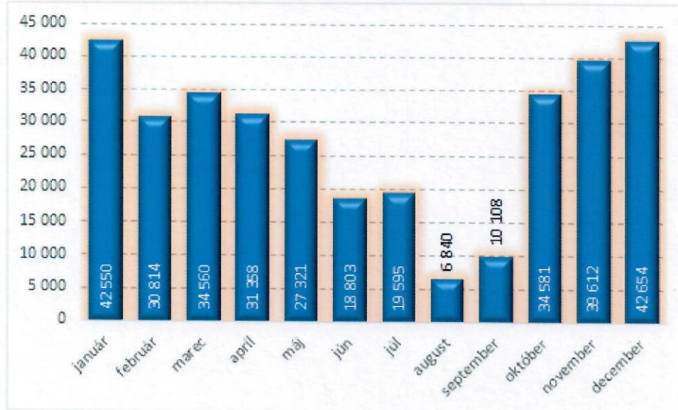
PPC Energy, a.s.: Výroba elektriny počas roka 2017 (v MWh)
